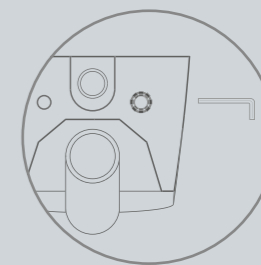
Fissaggio laterale nascosto Lateral fixing Seitliche Befestigung
